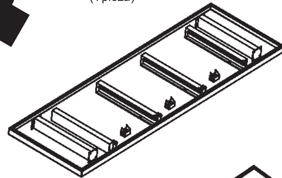
A Pieza de la parte superior del banco (1 pieza)
