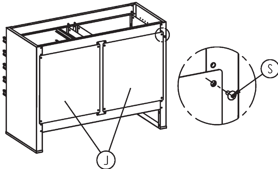
Ocho tornillos M5x12 (S)
